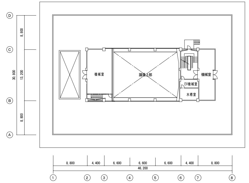
PH1階平面図
