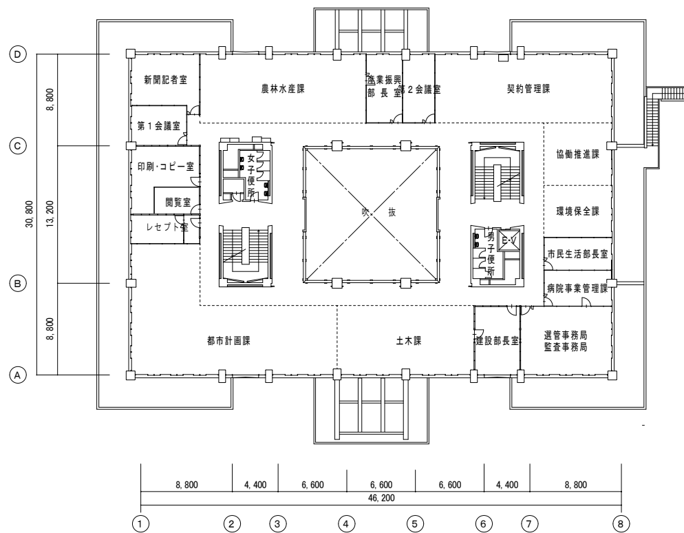
2階平面図
