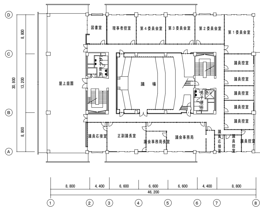
4階平面図
