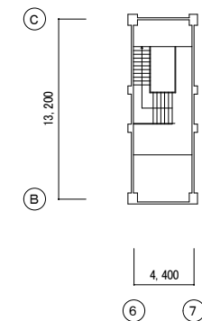
PH2階平面図
