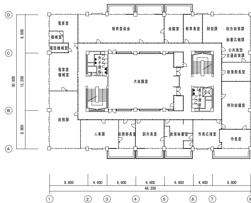
3階平面図
