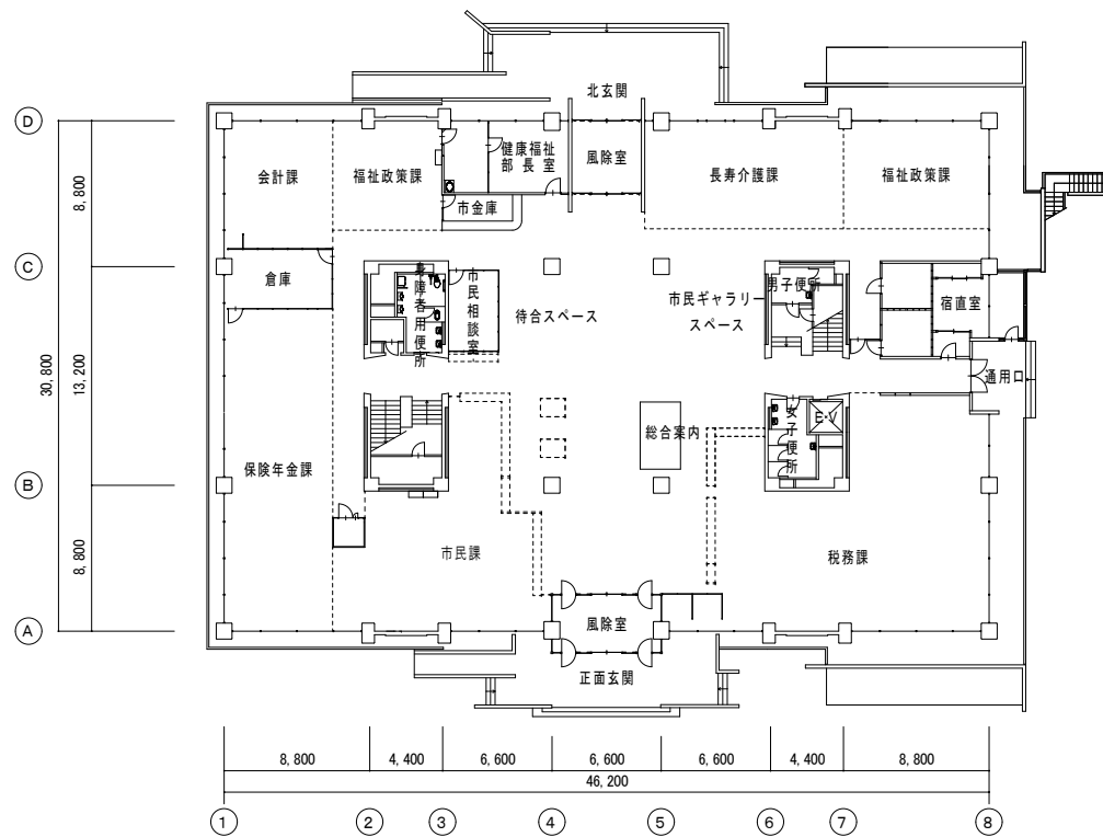
1階平面図
