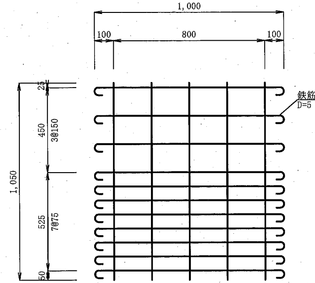
扉用メッシュ柵 S=1:20
