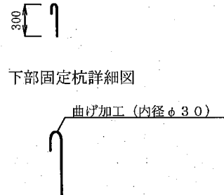
下部固定杭 (D10) S=1:50
