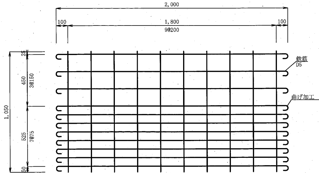
標準メッシュ柵 S=1:20
