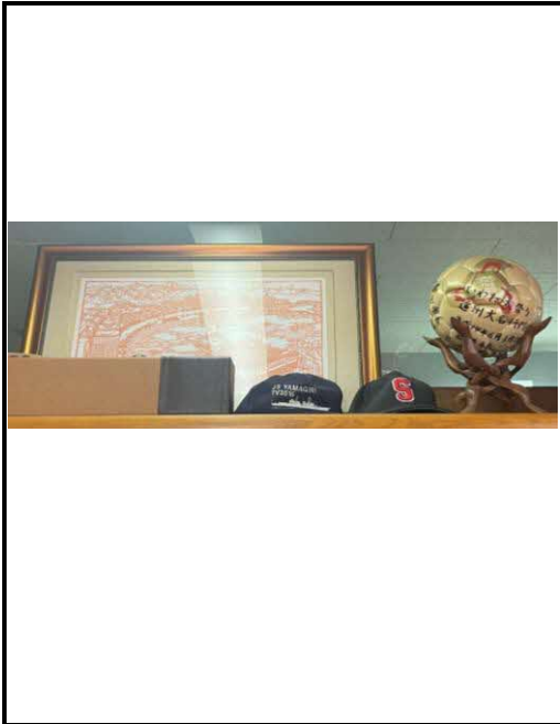
本庁舎 2階 市長応接室
